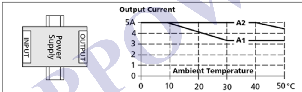
图 7-4-1 安装方向 D (水平安装方向)
