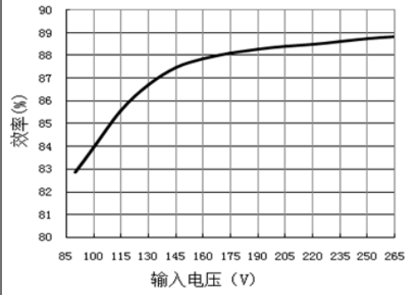
图 1-2-1 效率VS输入电压 at24V/5A, typ.
