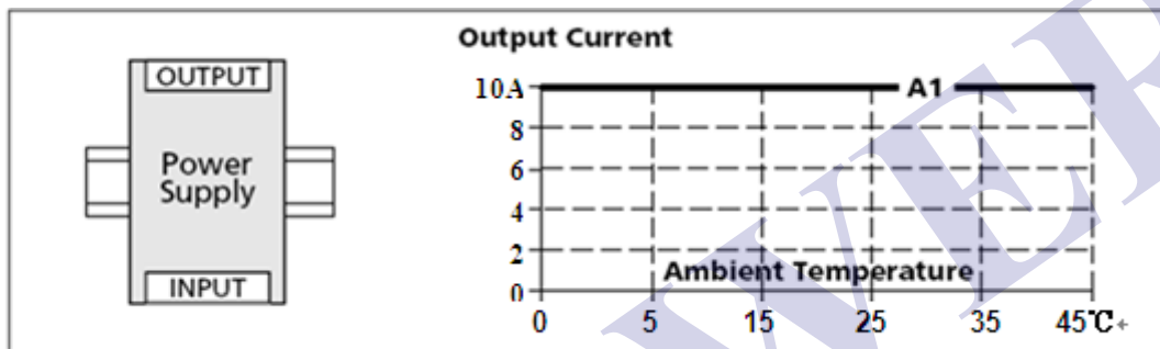
图 7-1 安装方向 A (标准安装方向)
