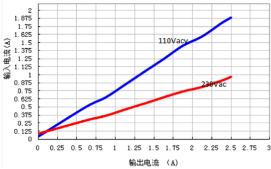
图 1-3-2 输入电流VS输出电流 @ 额定输出电压
