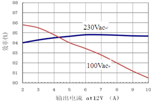
图1-1 效率VS输出电流 at12V, typ.
