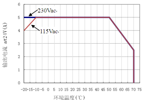
图 6-1-1 输出电流VS环境温度 at24V, typ.
