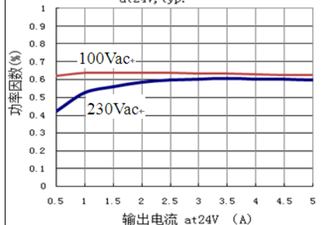
图 1-4-1 功率因数VS输出电流 at24V, typ.
