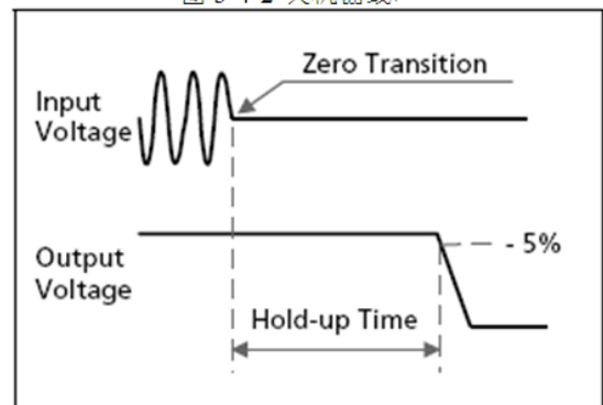
图 3-4-2 关机曲线
