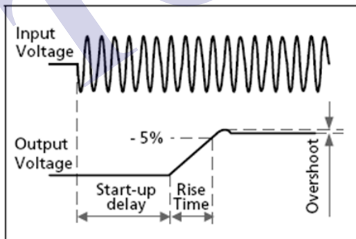
图 3-3 开机曲线
