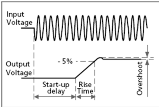
图 3-3-1 开机曲线
