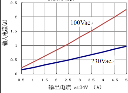
图 1-3-1 输入电流VS输出电流 at24V, typ.
