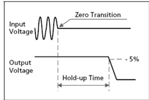
图 3-4 关机曲线
