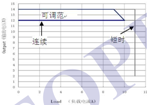
图 3-3 开机曲线
