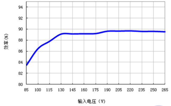
图 1-2-2 效率VS输入电压 @ 额定输出电压
