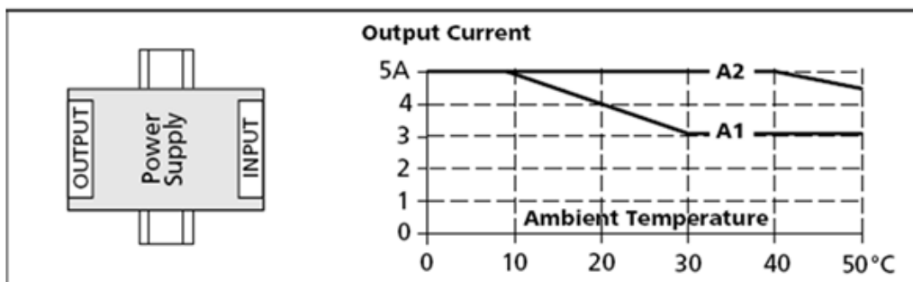
图 7-5-1 安装方向 E (水平安装方向)
