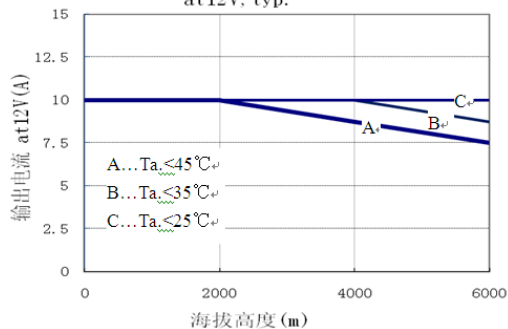
图6-2 输出电流VS海拔高度 at12V, typ.
