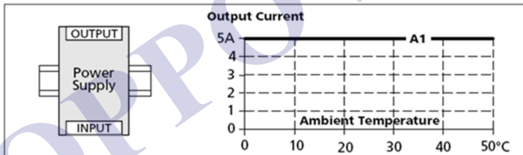
图 7-1-1 安装方向 A (标准安装方向)
