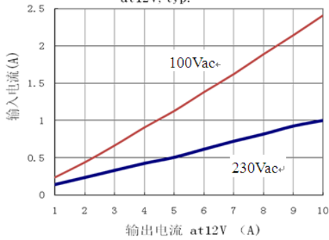
图1-3 输入电流VS输出电流 at12V, typ.
