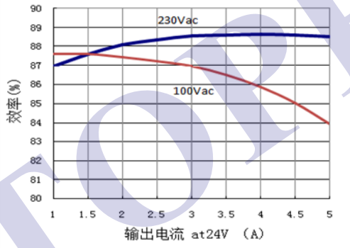
图 1-1-1 效率VS输出电流 at24V, typ.
