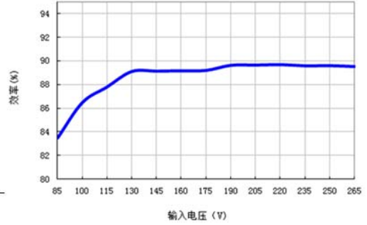
图 1-2-2 效率VS输入电压 @ 额定输出电压
