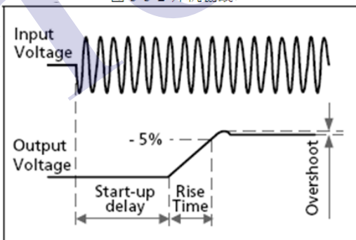
图 3-3-2 开机曲线
