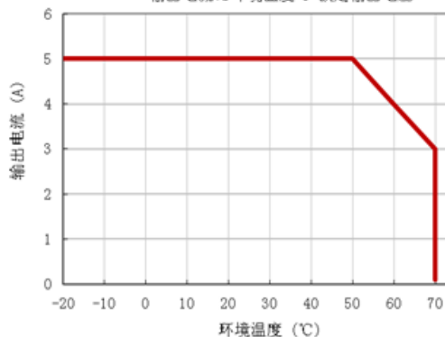
图 6-1-1 输出电流VS环境温度 @ 额定输出电压
