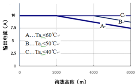
图6-2 输出电流VS海拔高度
