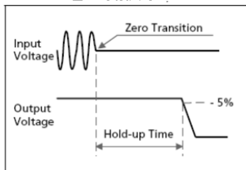
图 3-4 关机曲线
