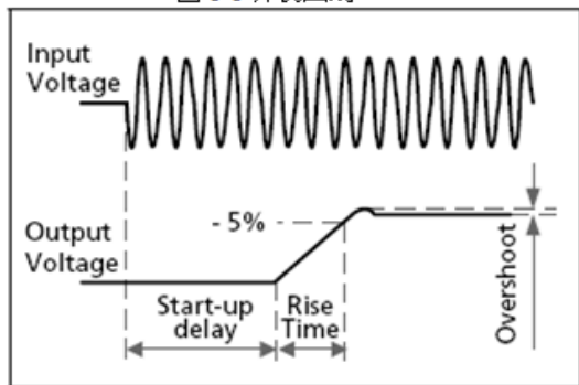
图 3-3 开机曲线
