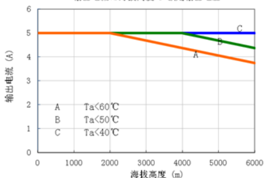
图 6-2-1 输出电流VS海拔高度 @ 额定输出电压
