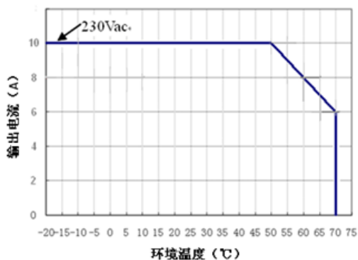
图6-1 输出电流VS环境温度 at 230Vac
